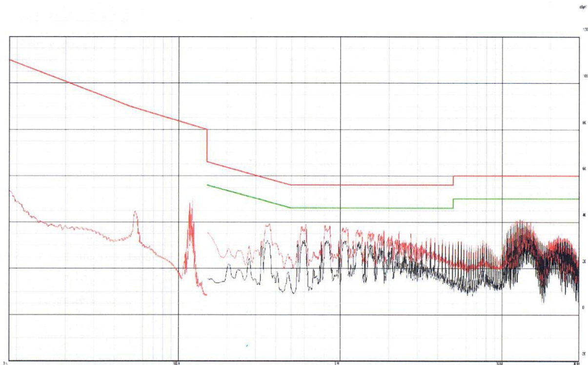
Obrázek C: Naměřené hodnoty na vodiči L v pásmu 9 kHz – 30 MHz – minimální výkon
